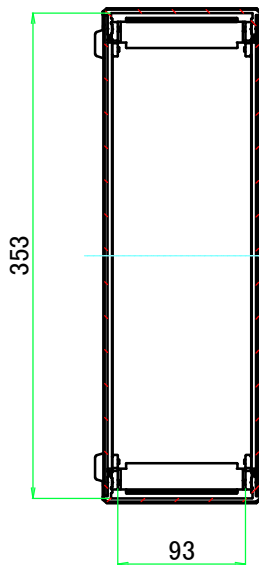
A-A ( 1 : 5.5 )
