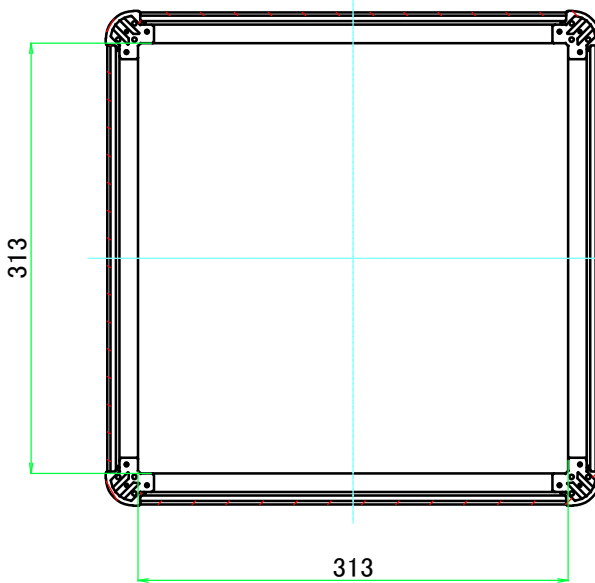
C-C ( 1 : 5.5 )
