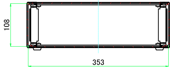
B-B ( 1 : 5.5 )
